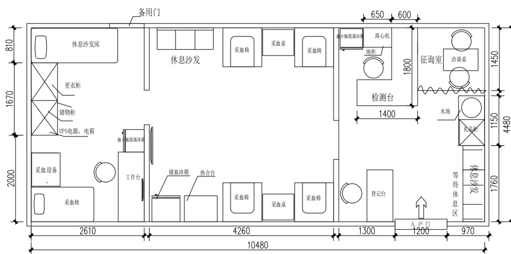
(5) 平面布置图
